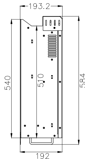
Widok od boku
