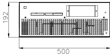
Widok od góry bez osłony
