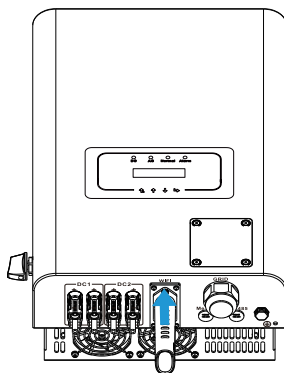
Rys. 5.13 Schemat instalacji rejestratora danych
