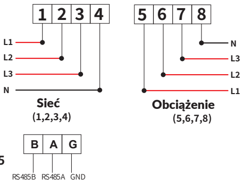
Rys. 7.3 Licznik Eastron
