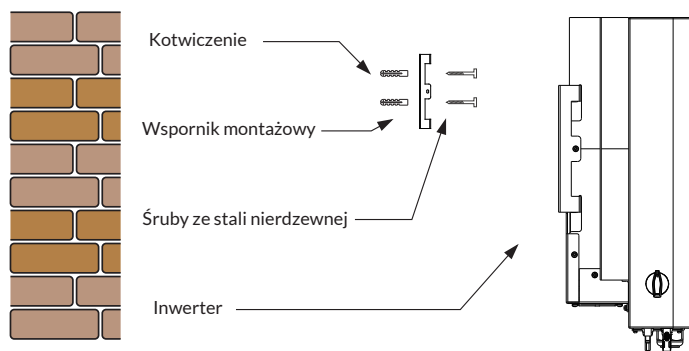
Rys. 4.4 Instalacja inwertera
