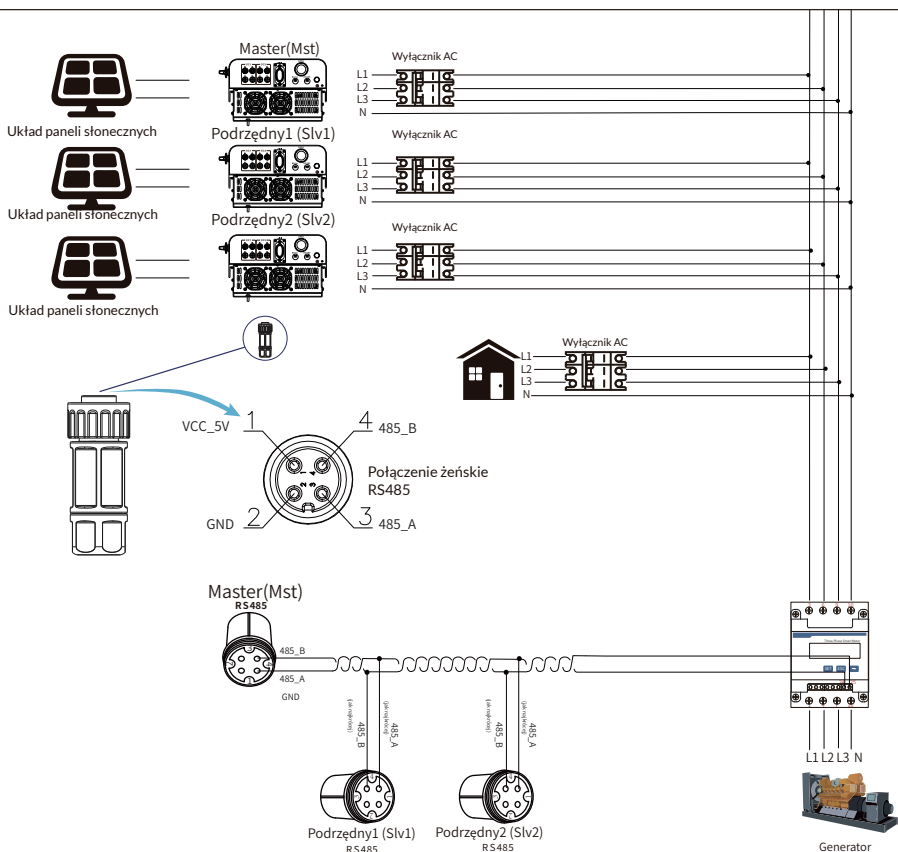
Rys. 7.29 Schemat połączenia CHNT (tabela przelotowa)
