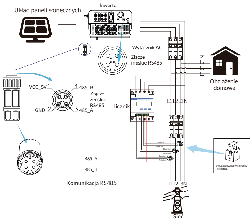
Rys. 7.14 Schemat połączeń licznika CHNT
