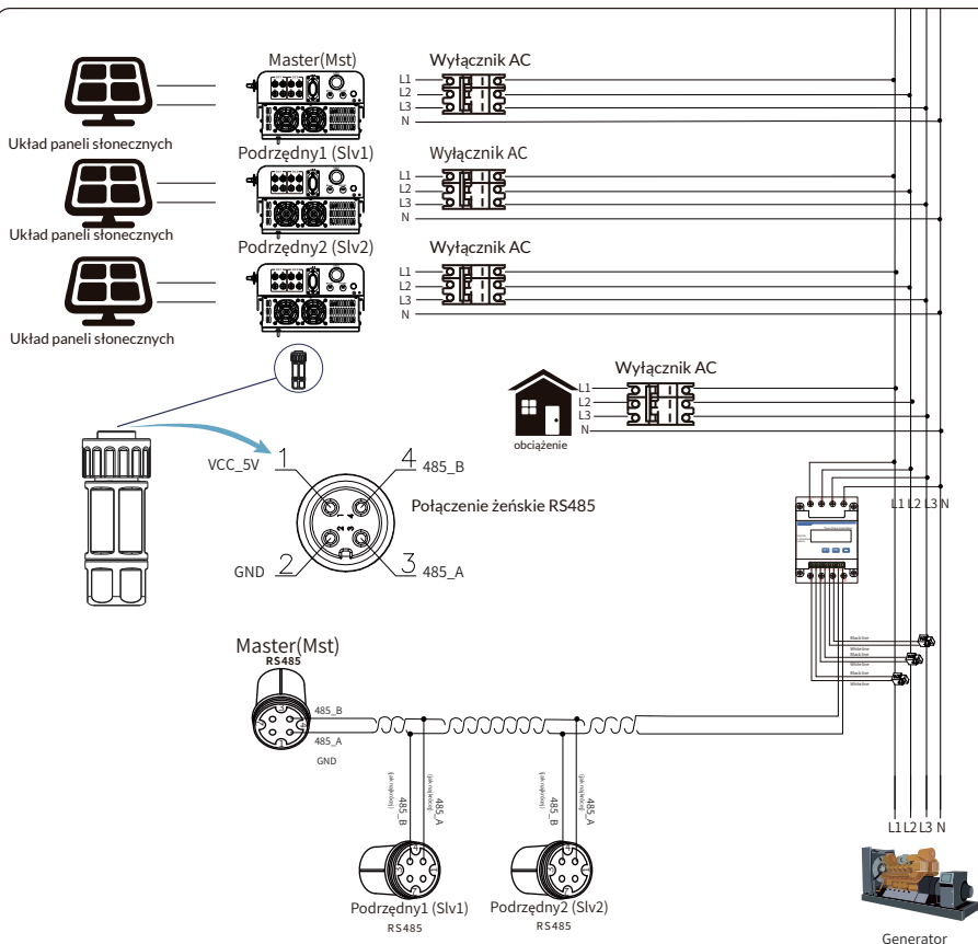
Rys. 7.33 Schemat połączenia CHNT (tabela przelotowa)
