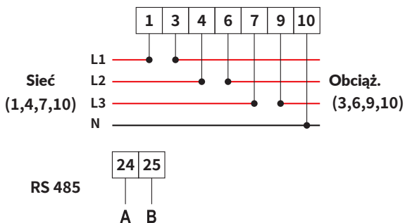
Rys. 7.28 Licznik CHNT
