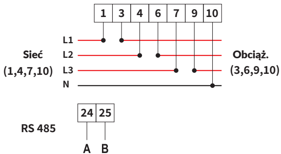
Rys. 7.9 Licznik CHNT
