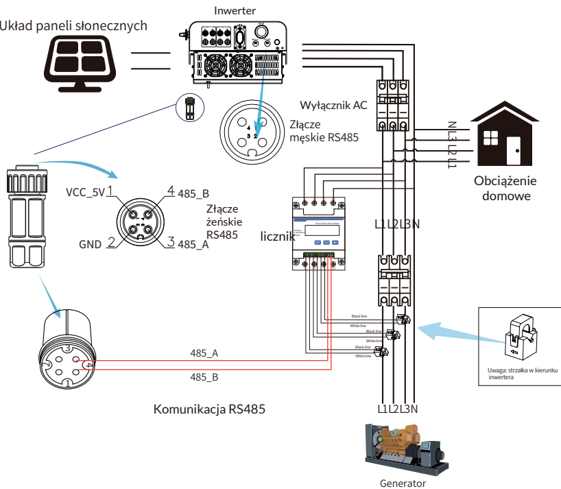
Rys. 7.16 Schemat połączeń licznika CHNT
