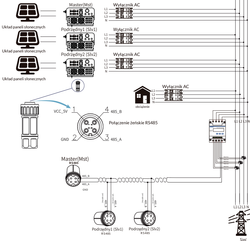
Rys. 7.31 Schemat połączenia CHNT (tabela przelotowa)
