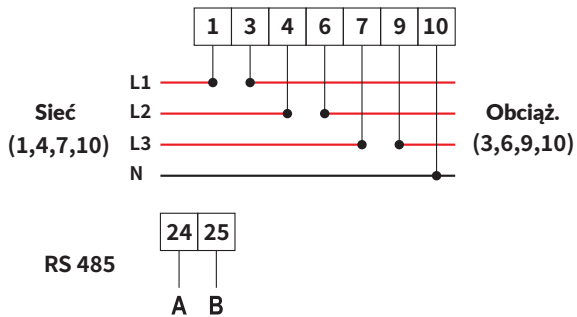
Rys. 7.11 Licznik CHNT
