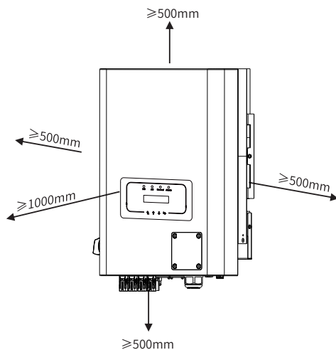
Rys. 4.3 Szczelina instalacyjna
