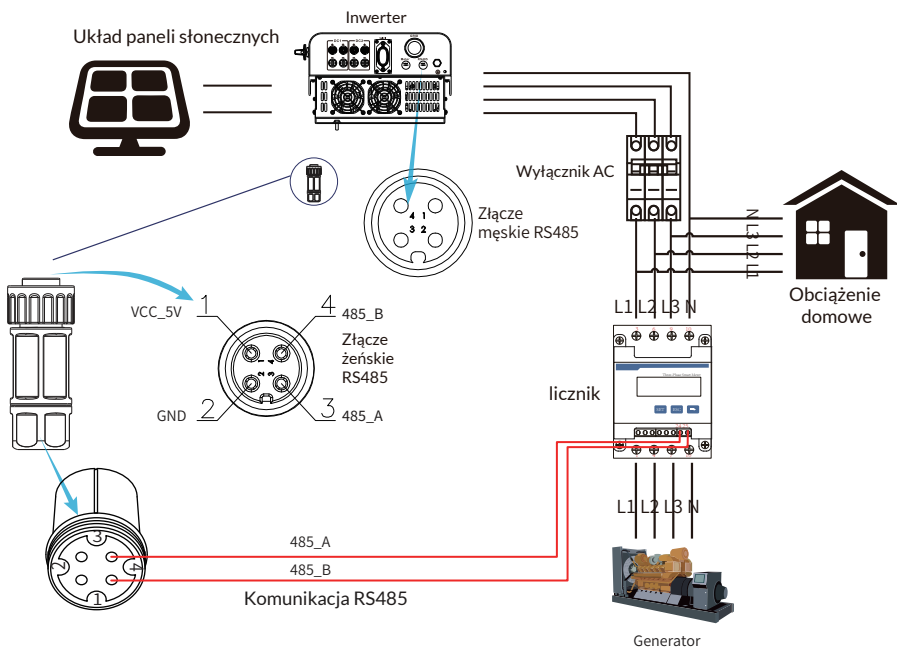
Rys. 7.12 Schemat połączeń licznika CHNT
