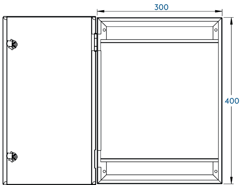
WIDOK PRZODU
