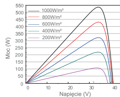
Krzywa moc-napięcie JAM72S30-540/MR
