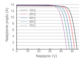
Krzywa prąd-napięcie JAM72S30-540/MR
