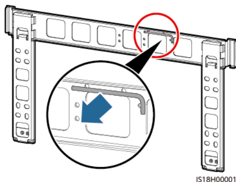
Rysunek 4-11 Wymywanie klucza Torx
