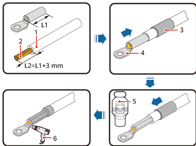
Rysunek 5-8 Zaciskanie zacisku DT
