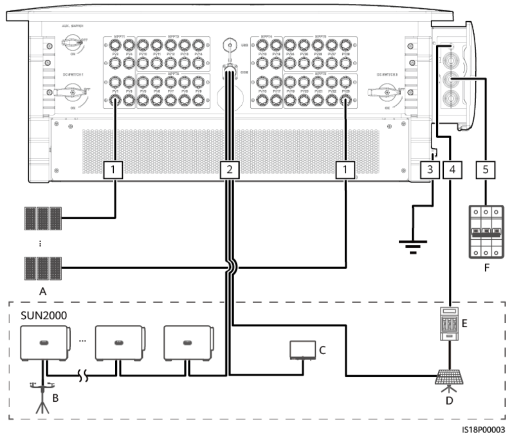
Rysunek 5-5 Podłączanie przewodów (należy skonfigurować komponenty przedstawione w zakreślowanym polu zgodnie z wymaganiami)
