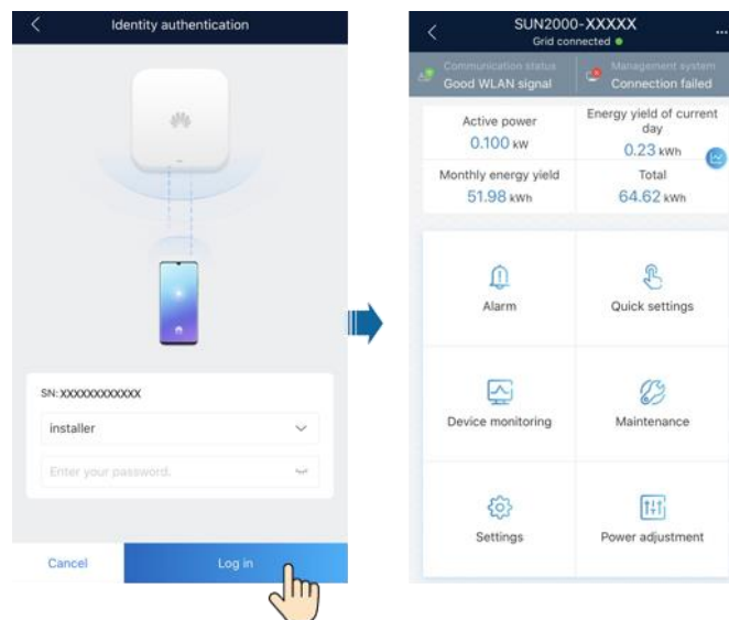
Rysunek 7-7 Logowanie
