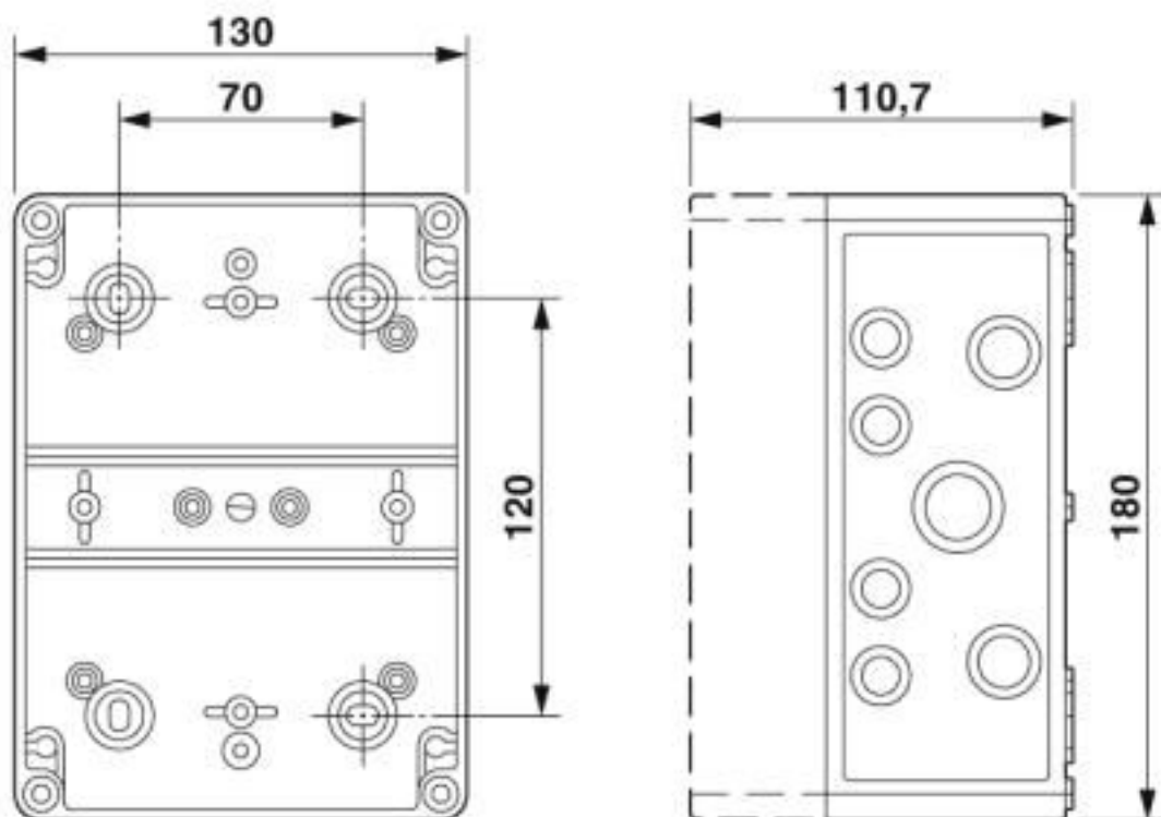
Rysunek wymiarowy
