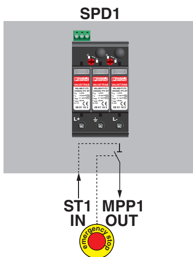
rysunek złączy
