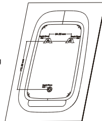
Installationsschablone X1
