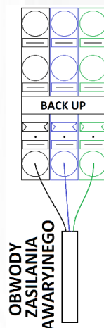
Rys.6 Blok zaciskowy przyłączenia zasilania awaryjnego wraz z przyłączonym obwodem zasilania awaryjnego.
