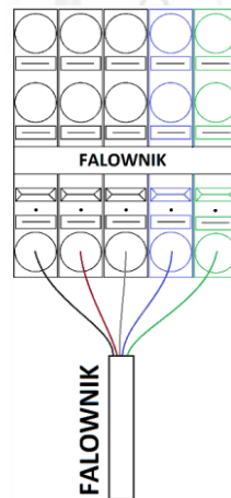
Rys. 5 Blok zaciskowy przyłącza falownika wraz z przyłączonym przewodem falownika.
