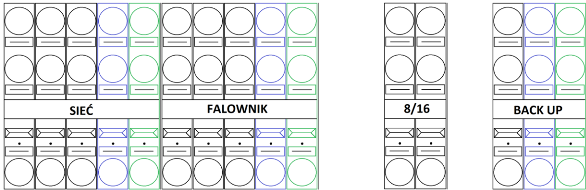
Rys. 3 Blok zaciskowy obwodów zasilania oraz sterowania.
