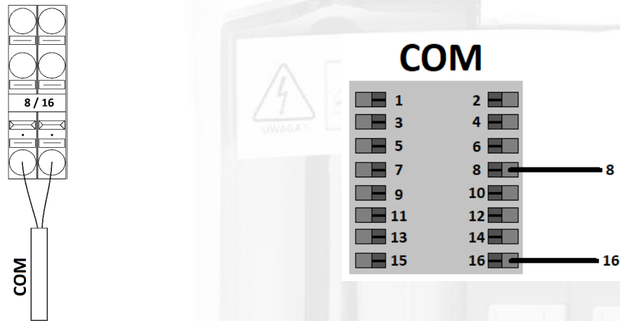
Rys. 7 Blok zaciskowy przyłącza komunikacji wraz z sposobem podłączenia złącza COM w falowniku.
