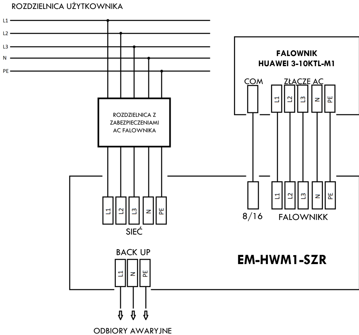
Rys. 2 Schemat przyłączeniowy.
