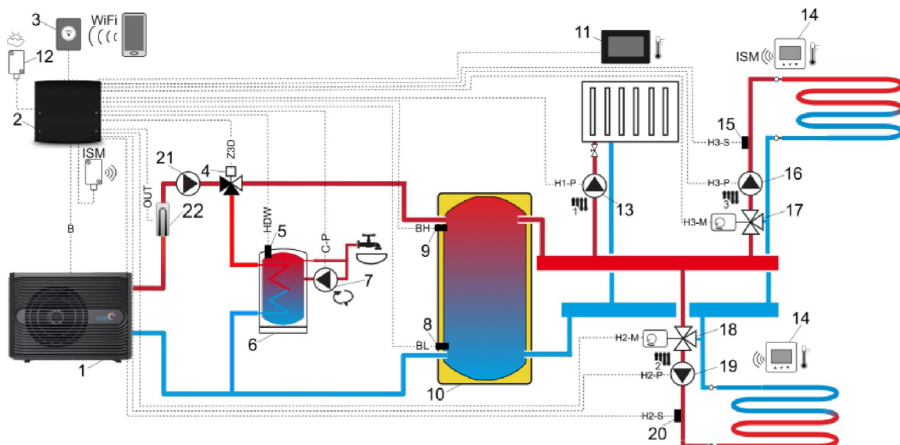
Schemat z buforem ciepła i zasobnikiem CWU 2 : 1 – pompa ciepła, 2 – regulator, 3 – moduł internetowy, 4 – zawór 3-drogowy, 5 – czujnik temp. zasobnika CWU, 6 – zasobnik CWU, 7 – pompa cyrkulacji, 8 – dolny czujnik temp. bufora, 9 – górny czujnik temp. bufora, 10 – bufor ciepła, 11 – panel sterujący z funkcją termostatu pokojowego, 12 – czujnik temp. zewnętrznej (pogodowy), 13 – pompa mieszacza 1, 14 – bezprzewodowy termostat pokojowy, 15 – czujnik temp. mieszacza 3, 16 – pomp mieszacza 3, 17 – siłownik mieszacza 3, 18 – siłownik mieszacza 2, 19 – pompa mieszacza 2, 20 – czujnik temp. mieszacza 2, 21 – pompa CWU, 22 – grzałka przepływowa.
