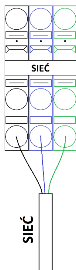
Rys.3 Blok zaciskowy sieci wraz z przyłączonym zasilaniem rozdzielnicy.
