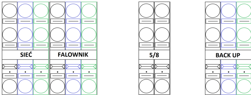
Rys.2 Blok zaciskowy obwodów zasilania oraz sterowania.
