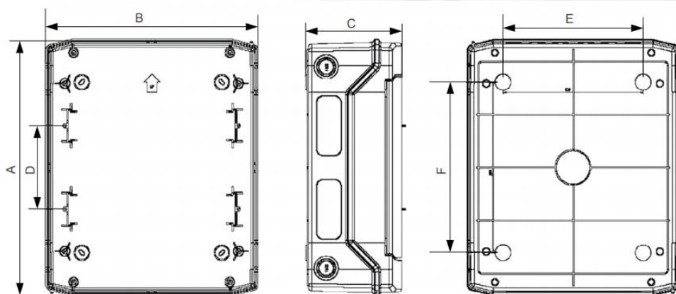
Rys.1 Wymiary obudowy.
