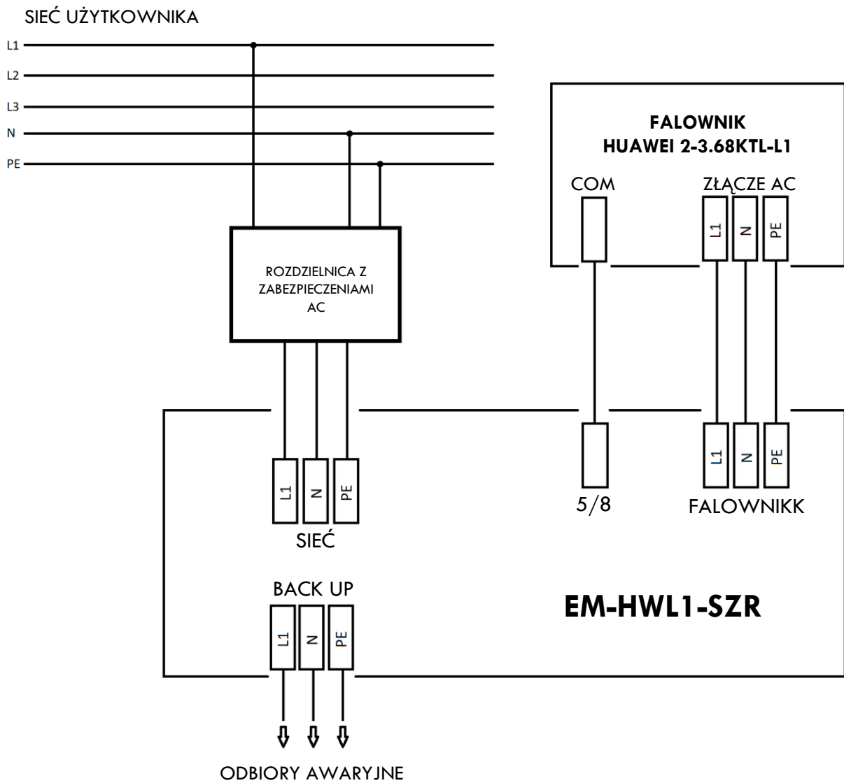
Rys.1 Schemat przyłączeniowy.
