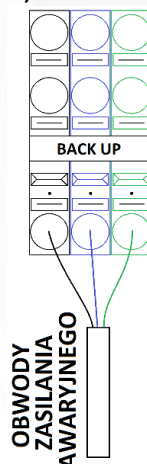
Rys.5 Blok zaciskowy przyłączenia zasilania awaryjnego wraz z przyłączonym obwodem zasilania awaryjnego.
