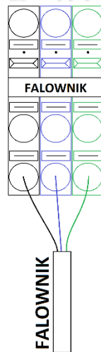
Rys.4 Blok zaciskowy przyłączenia falownika wraz z przyłączonym przewodem falownika.
