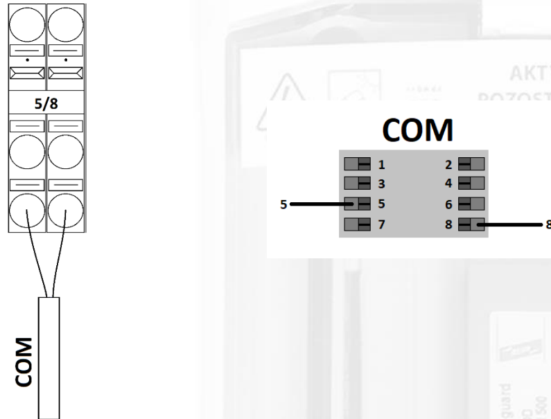
Rys.6 Blok zaciskowy przyłączenia komunikacji wraz z sposobem zarobienia złącza COM w falowniku.
