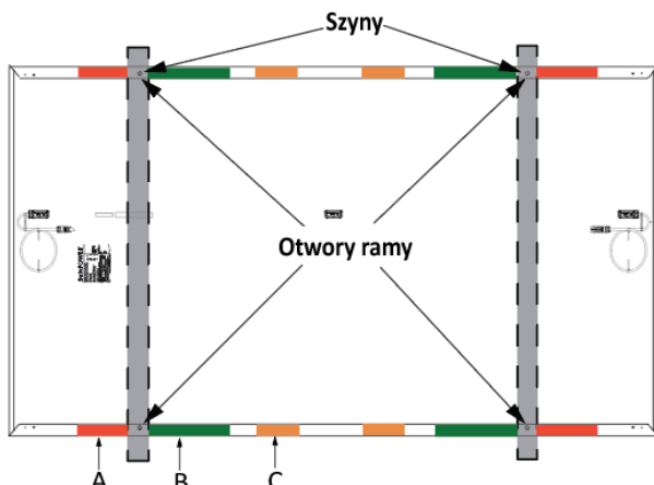
Rysunek 4: Lokalizacja stref montażowych dla modułów Performance
