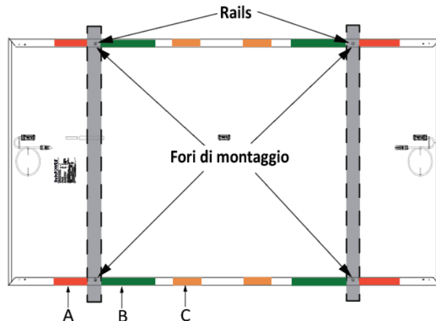
Figura 4: Zone di montaggio delle delle pinze o morsetti per il modulo Performance UPP
